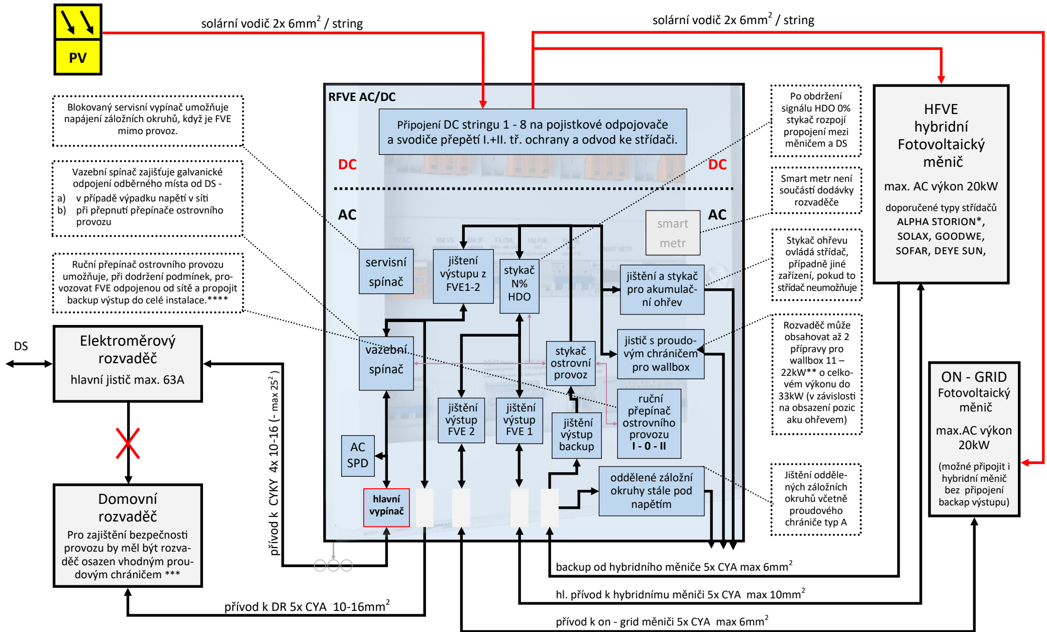
Přehledové schéma je platné pro AC-DC model MAX 63A KAVOJ RFVE-O-Nx-1-x-x-63-xxxV-0x
