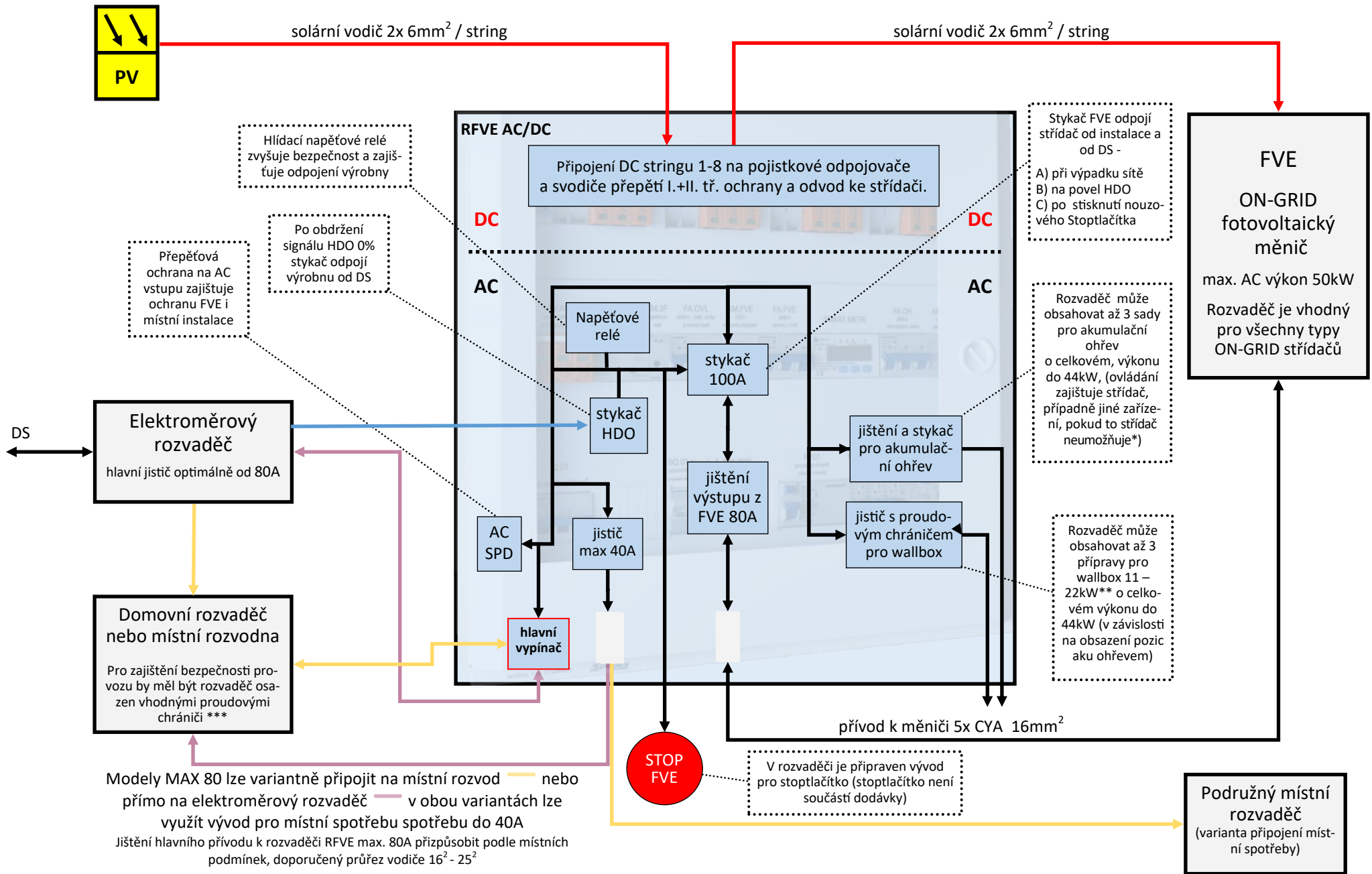
Přehledové schéma je platné pro modely MAX 80A KAVOJ RFVE-O-xx-1-x-x-80-xxxV-0x
