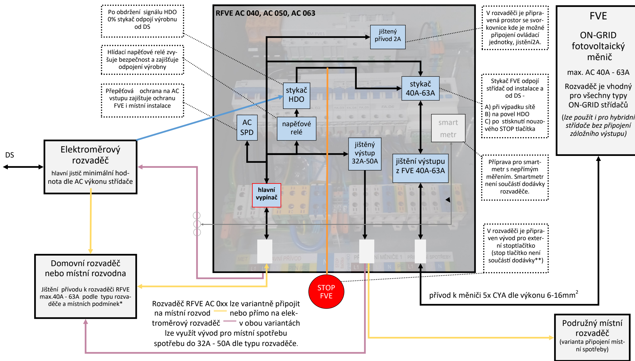
Přehledové schéma je platné pro modely KAVOJ RFVE AC 040, AC 050, AC 063
