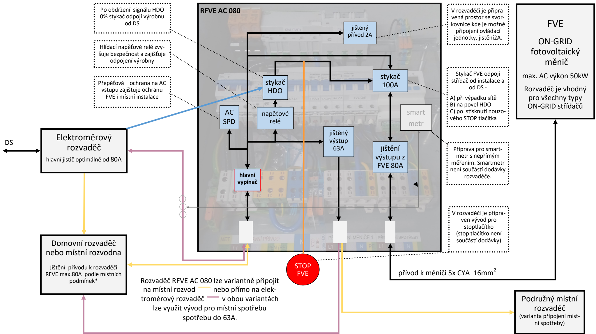
Přehledové schéma je platné pro modely KAVOJ RFVE AC 080
